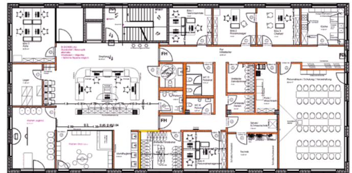
ERDGESCHOSS
